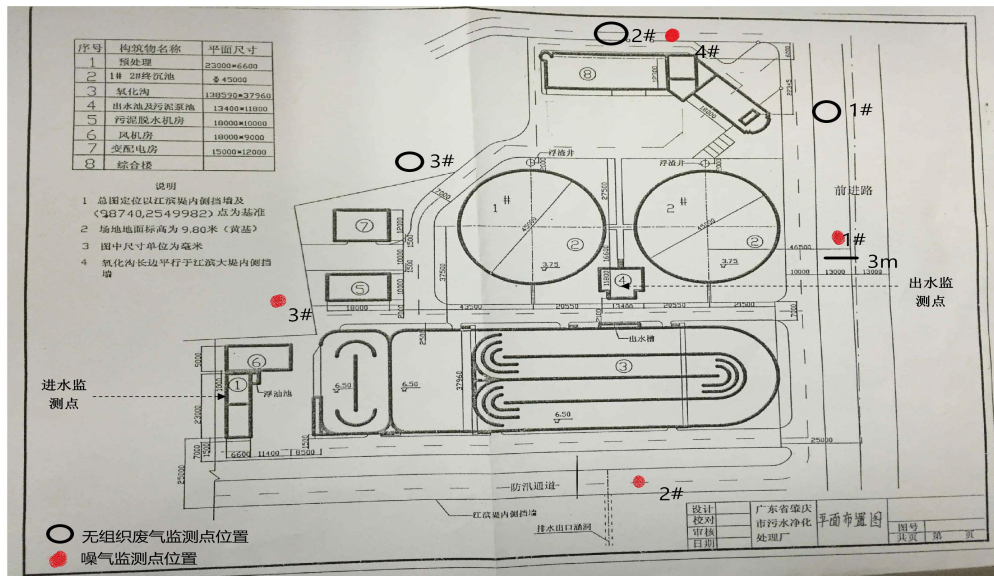
图 2：第一污水处理厂平面布置及监测点位分布图
