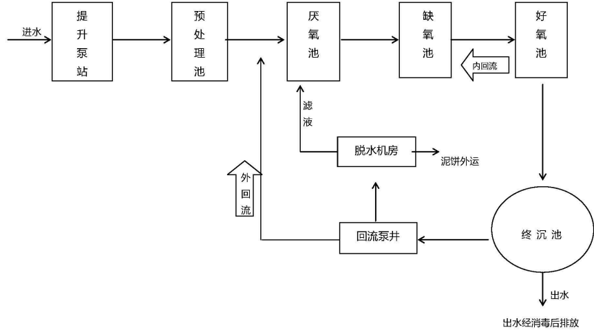
一厂工艺流程图
