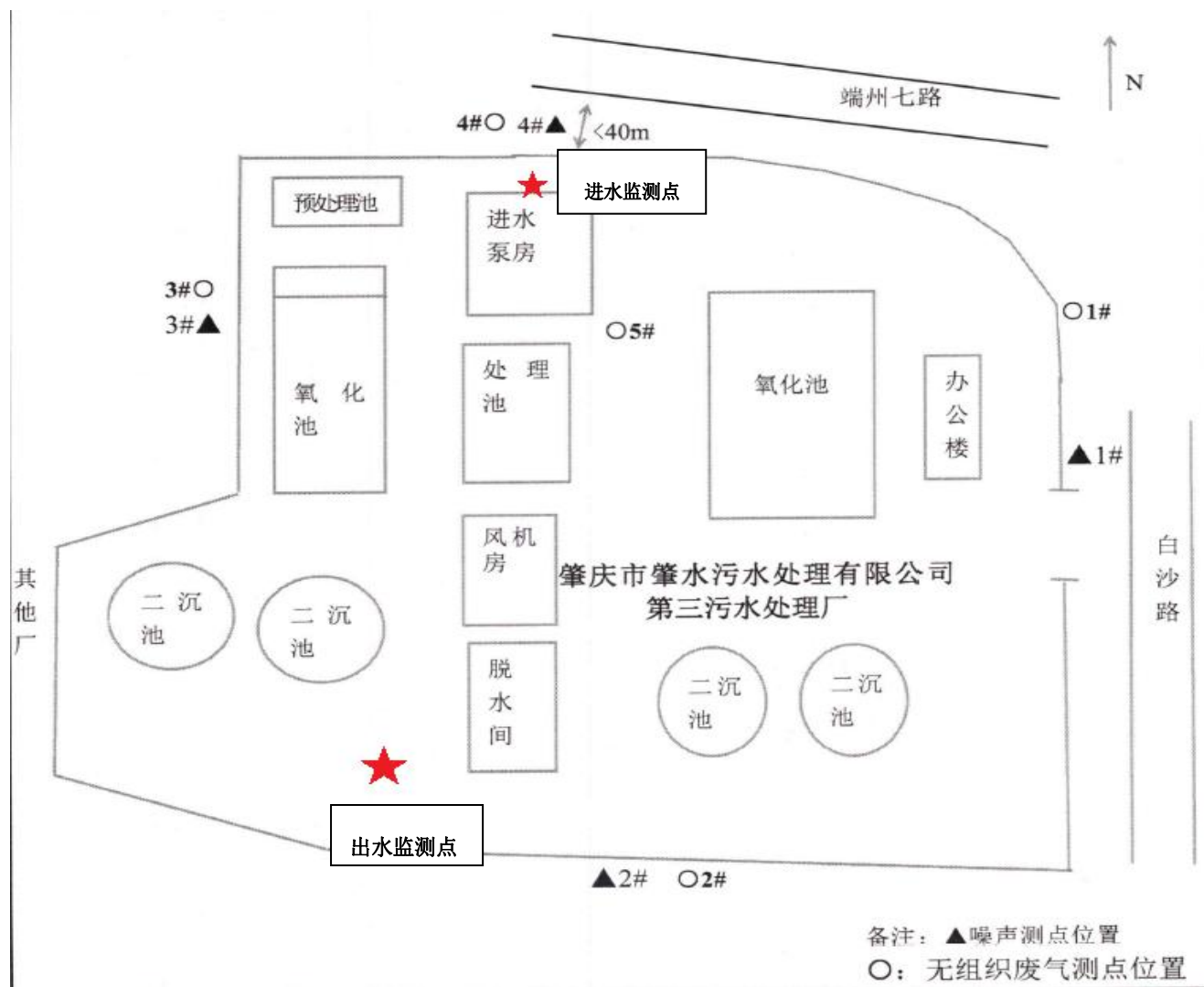
图 2 全厂平面布置及监测点位分布图
