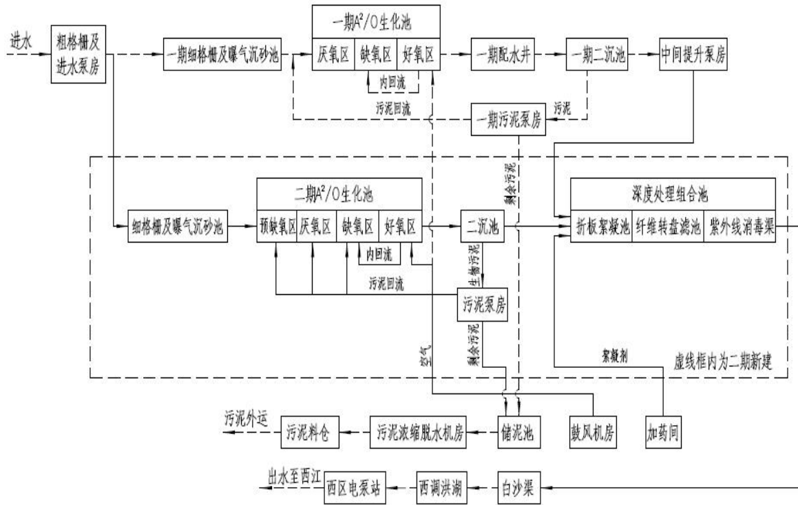
图 1 污水处理工艺流程示意图
