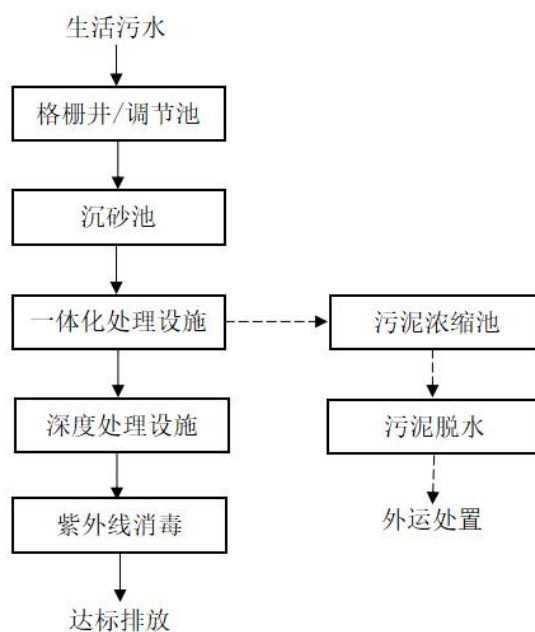
图 1 德庆肇水环保有限责任公司官圩镇污水厂工艺流程图
