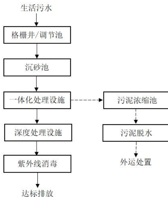
图 1 德庆肇水环保有限责任公司播植镇污水厂工艺流程图
